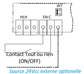
Schéma #6
