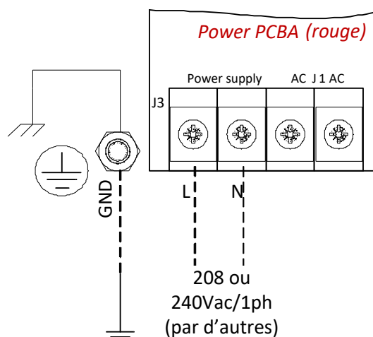
Figure 16 – Connexion de l'alimentation électrique
