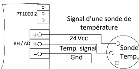
Schéma #4
