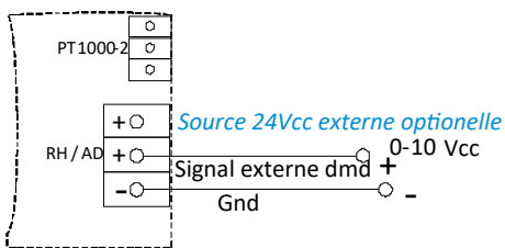
Schéma #4
