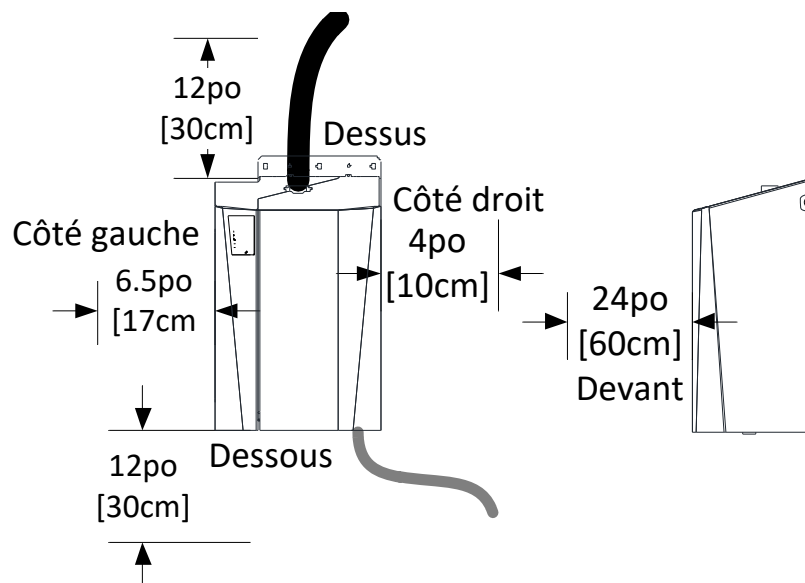
Figure 5 – dégagements conseillés
