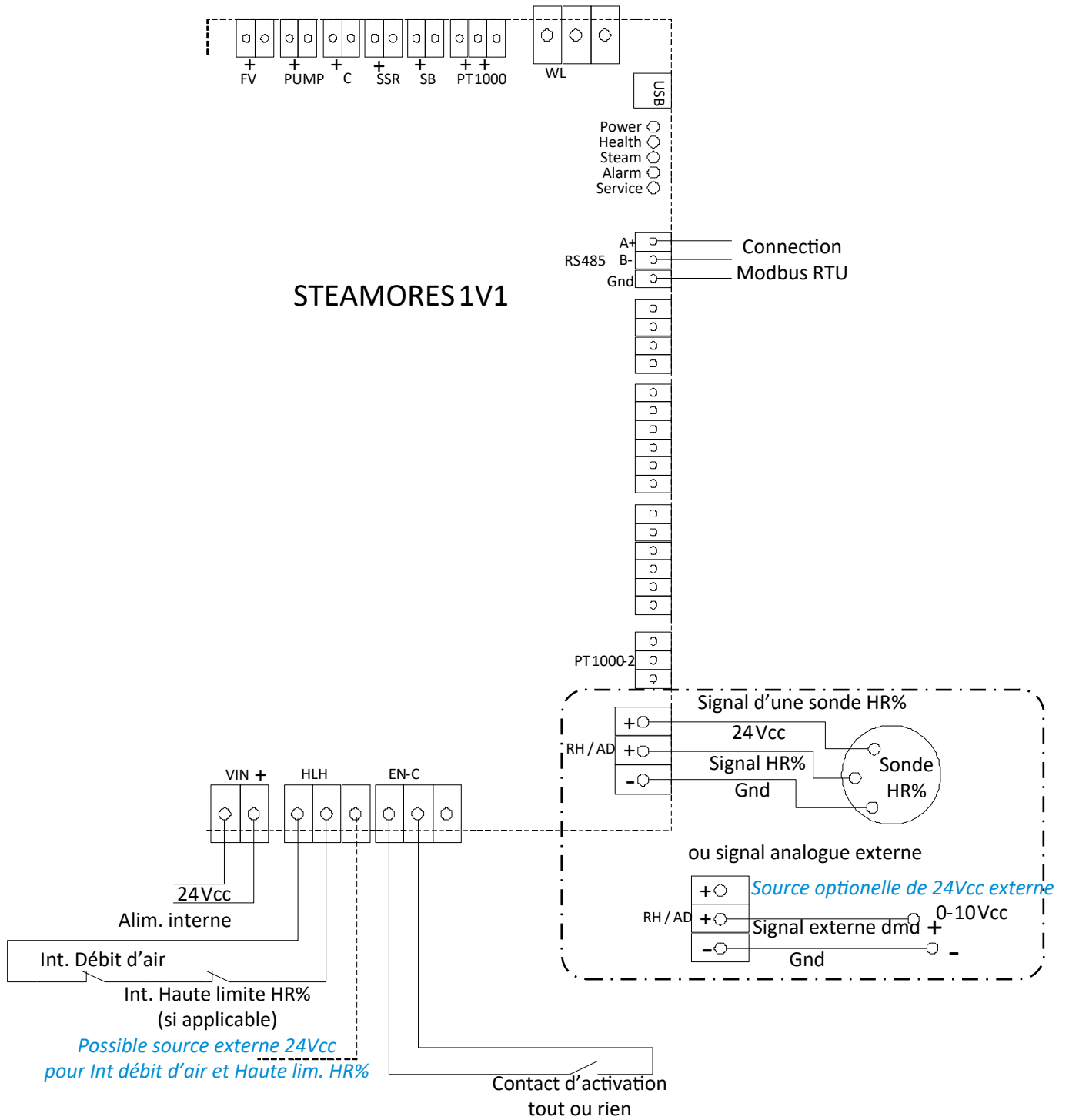
Figure 17 – Connexions des entrées de contrôles
