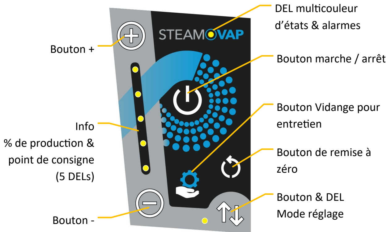
Figure 18 – Panneau tactile du RES
