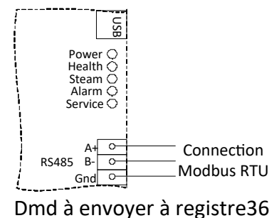
Schéma #6
